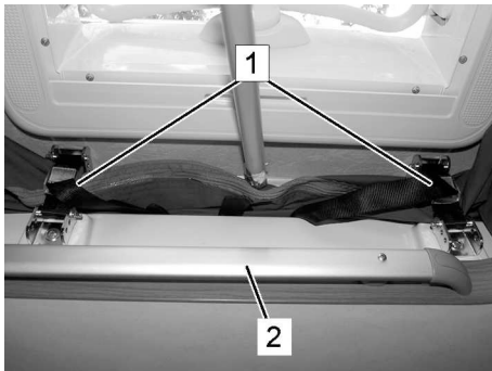
Fig. 147 : Déplier le toit ouvrant
