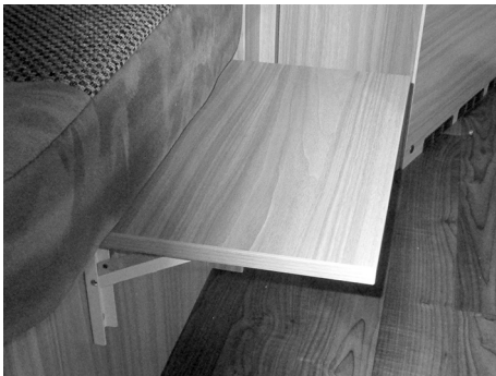
Fig. 144 : Console pliante servant de rallonge de lit
