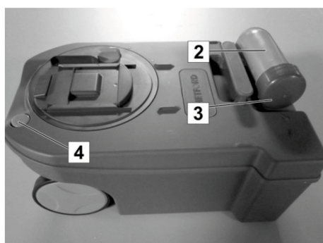
Fig. 158 : Vidange de la cassette WC
