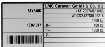
Fig. 1 : Plaque signalétique
