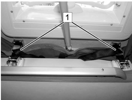
Fig. 151: Fermetures de toit (1)
