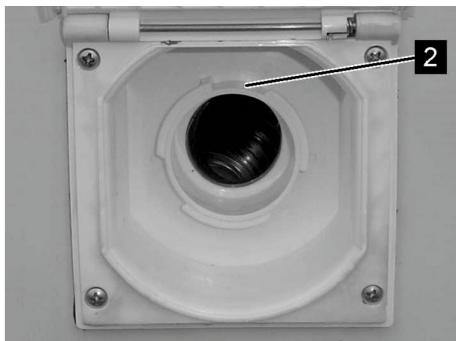
Fig. 102 : manchon de remplissage d'eau fraîche, ouvert
