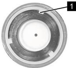
Fig. 101 : bouchon à visser, côté intérieur
