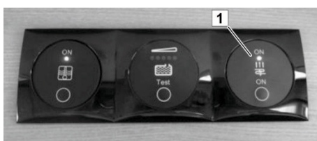
Fig. 133 : Boutons Marche/Arrêt du chauffage au sol
