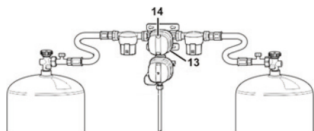
Fig. 113 : Kit détenteur
