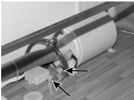
Fig. 97: Chauffe-eau TRUMA et vannes de vidange d'eau
