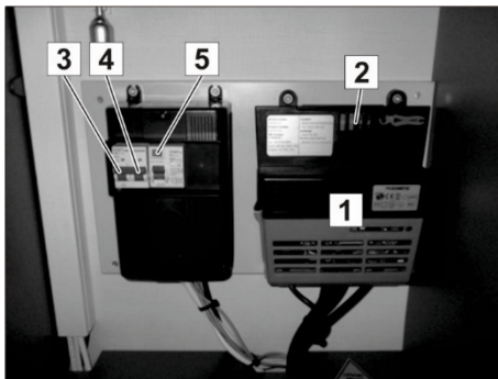
Fig. 67 : Transformateur (bloc d'alimentation) (1) et disjoncteurs
